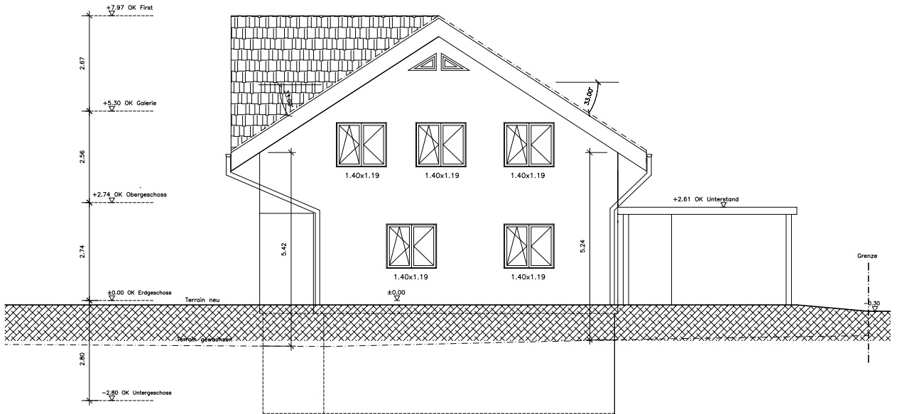
OST FASSADE
