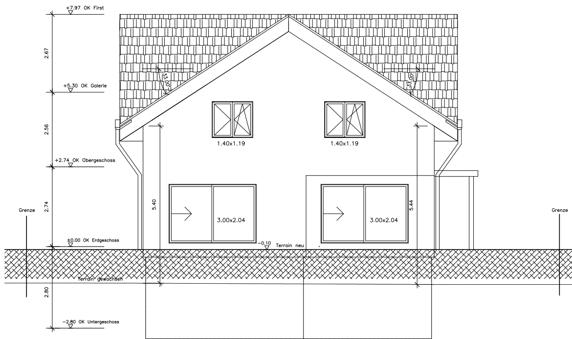
SÜD FASSADE
