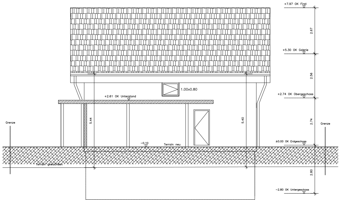
NORD FASSADE
